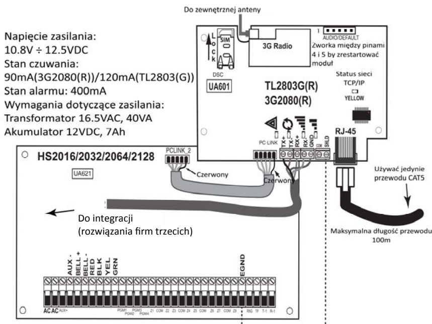
Rysunek 3 Diagram połączeń elektrycznych
