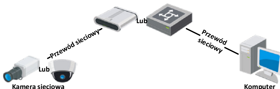
Rysunek 2–2 Połączenie przy użyciu przełącznika lub routera
