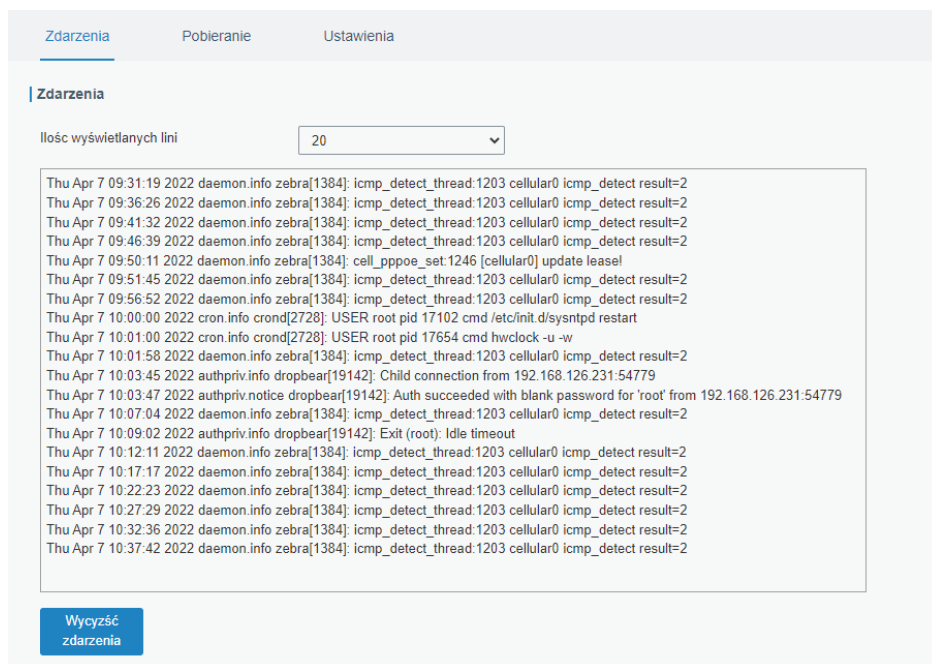
Obrázok 4.119 Funkcia udalostí
