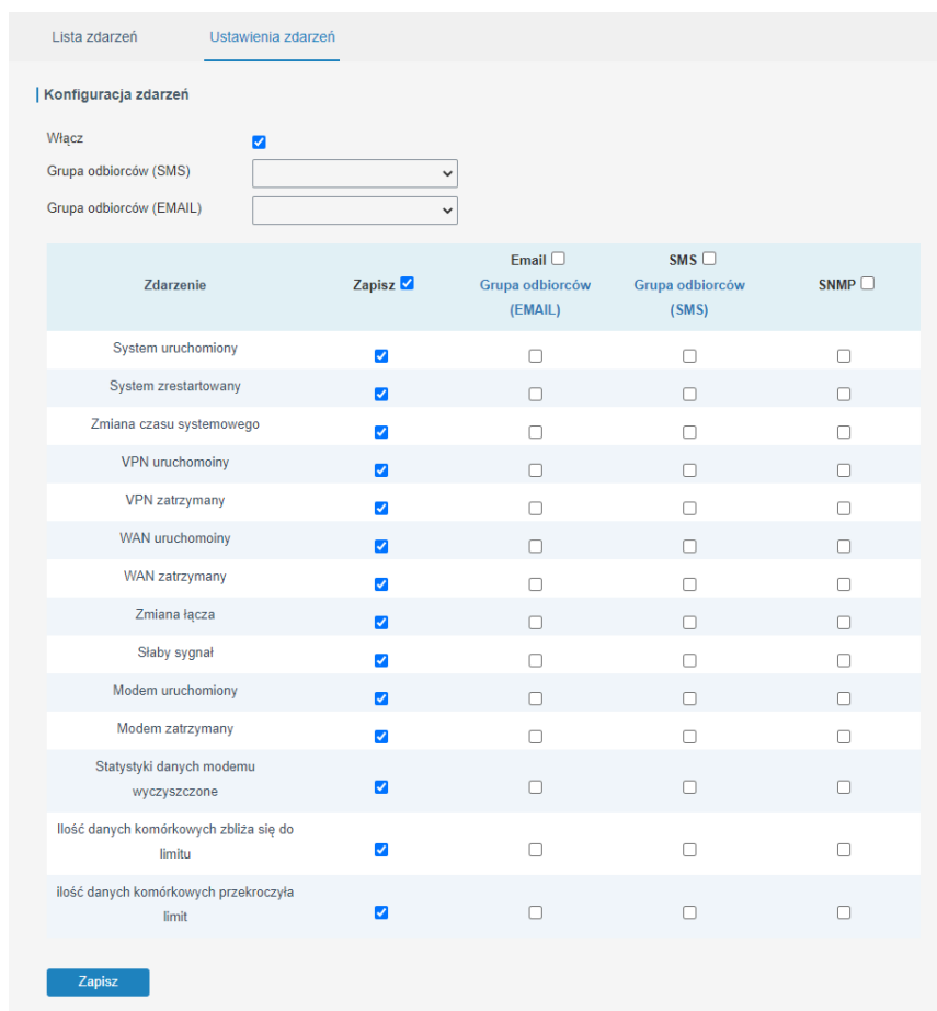
Obrázok 4.112 Konfiguracja záložky Nastavenia udalostí
