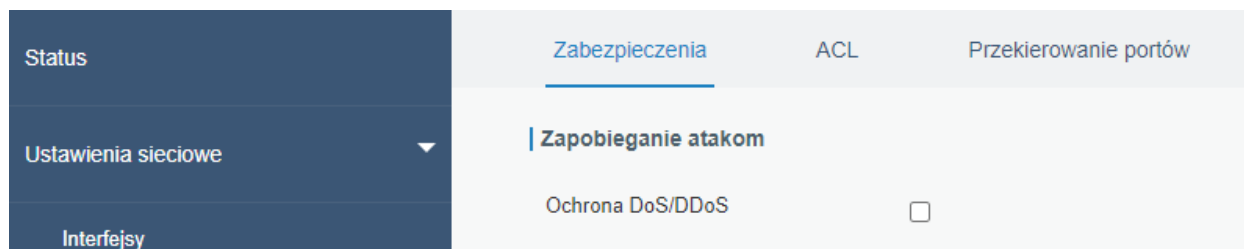
Obrázok 4.30 Ochrana DoS/DDoS
