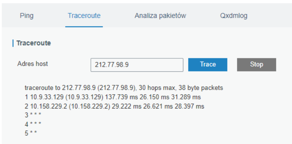
Obrázok 4.114 Funkcia Traceroute
