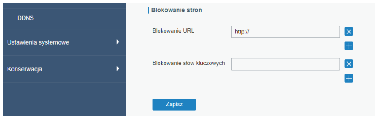
Obrázok 4.32 Blokowanie stránok
