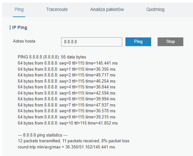
Obrázok 4.113 Funkcia Ping
