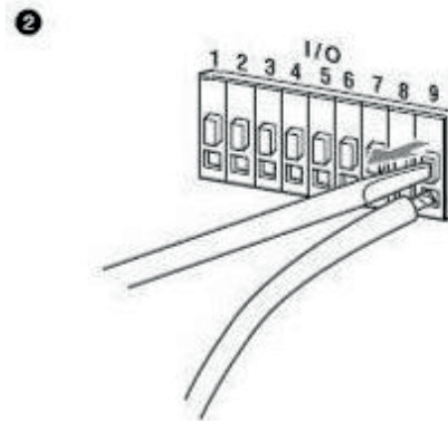
Nákres 8-5 Odpájanie kábla
