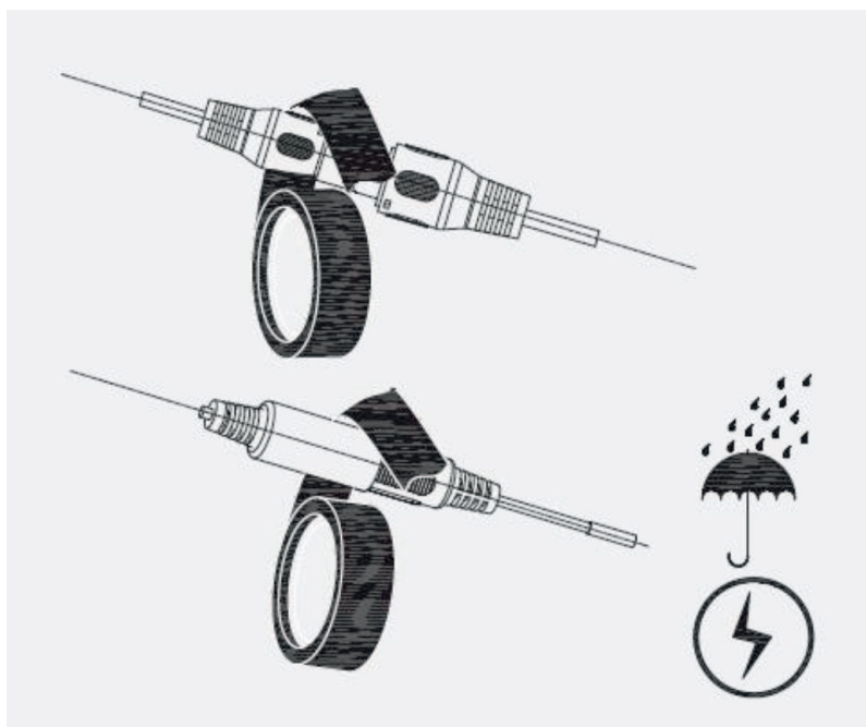
Rysunek 10-2 Środki wodoszczelne
