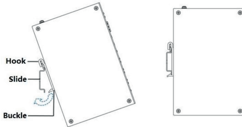
Nákres 3-1 Inštalácia
