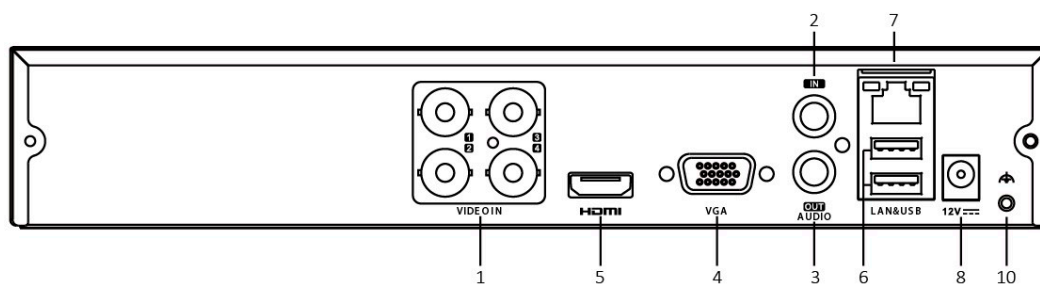
Rysunek 1–5 Panel tylny BCS-B-XVR0401
