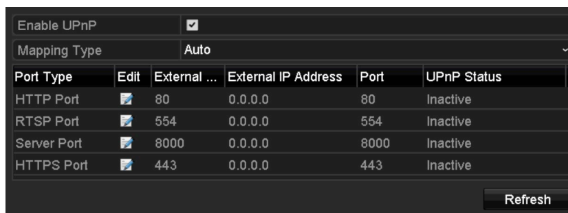
Rysunek 11–8 Ustawienia funkcji UPnP™
